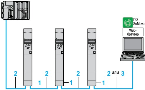
Modicon M340 (4)
